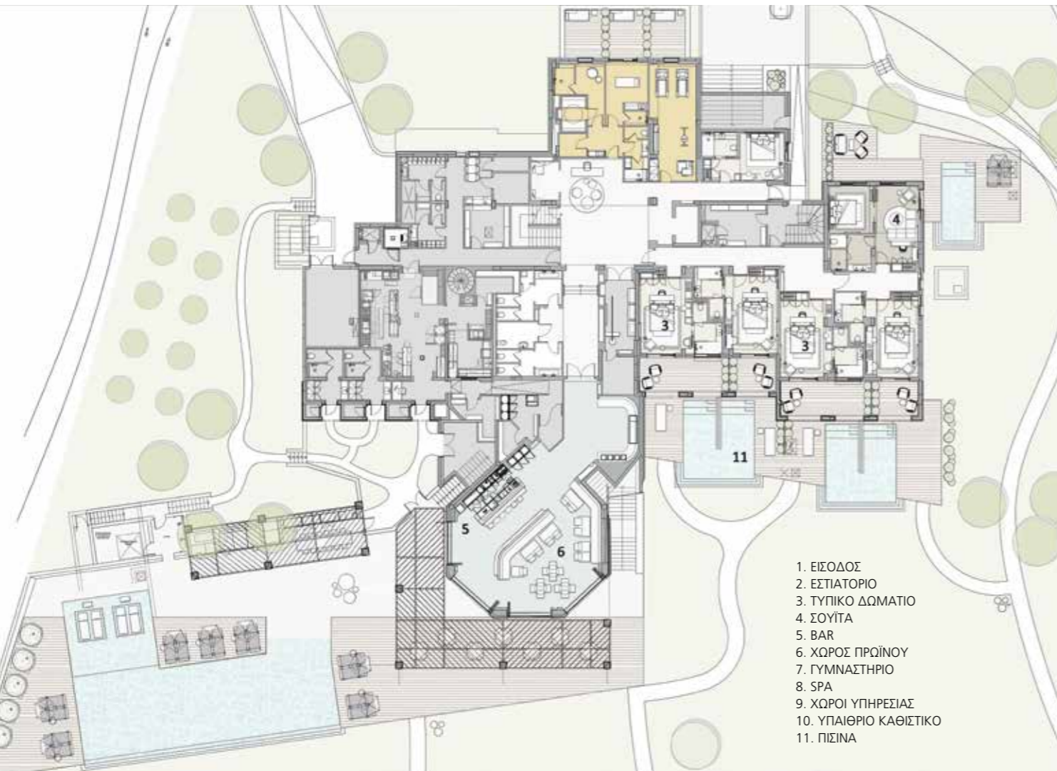
κάτοψη ισογείου
